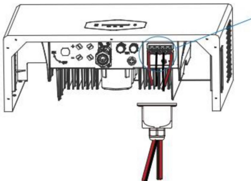
HÁLÓZAT EPS fogyasztó
